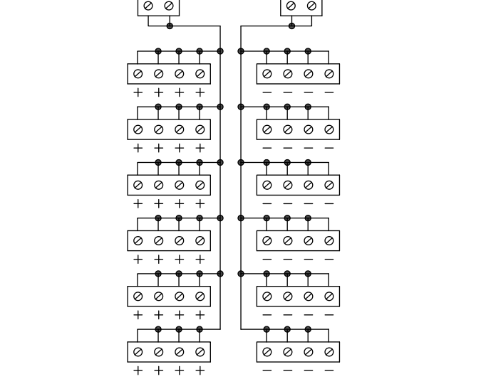
接 线 图
