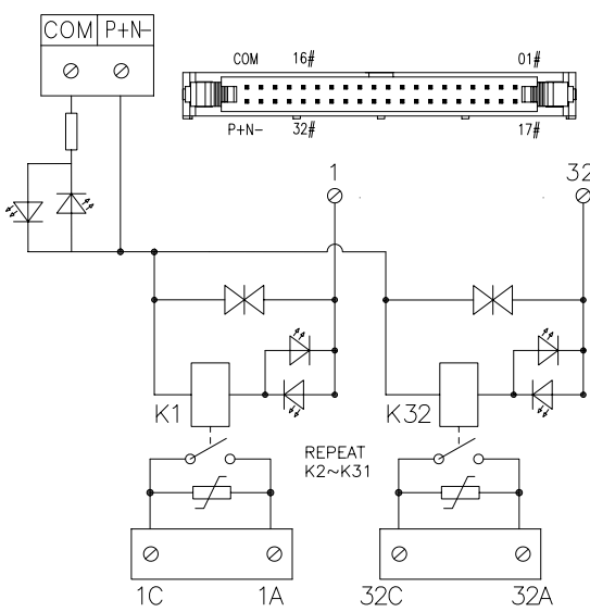
接 线 图
