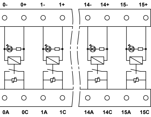
接 线 图
