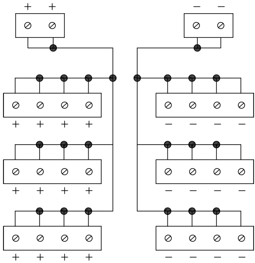
接线图
