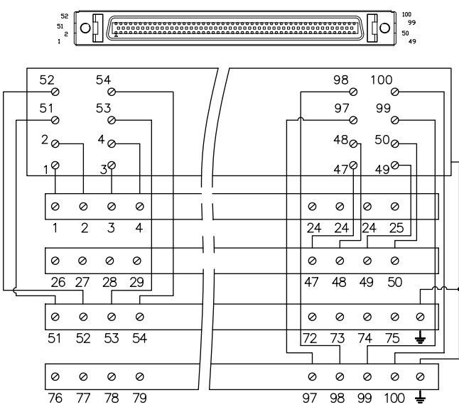
接 线 图
