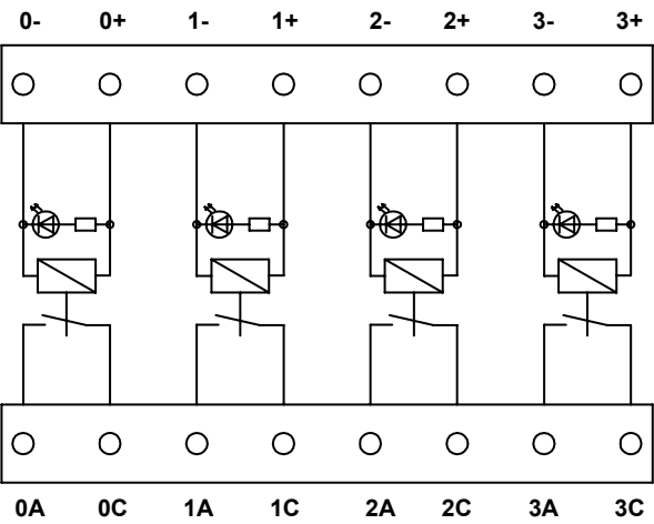
接 线 图
