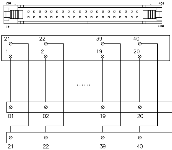
接 线 图
