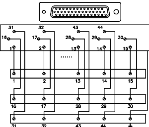
0241-C2XX 接線圖
