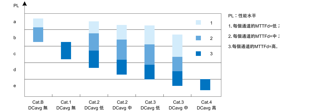
PL 和每個通道的類別、DCavg 和 MTTFd 的關係
