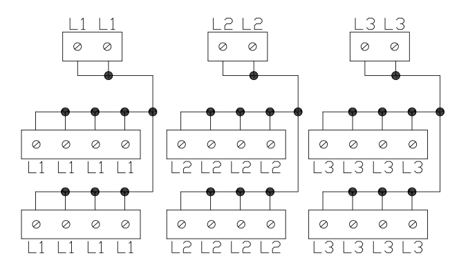
接線圖
