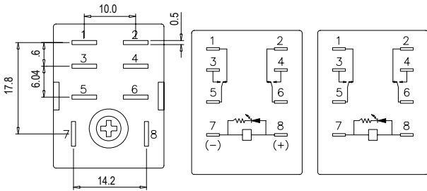
DC 接線圖 AC 接線圖
