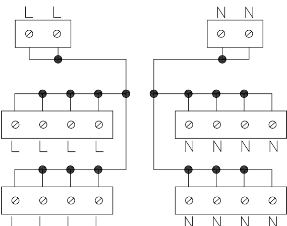
接線圖
