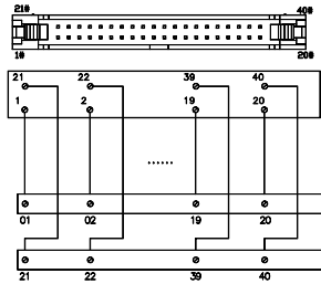
0241-C1XX 接線圖
