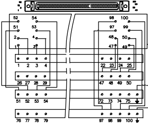
0241-C3XX 接線圖
