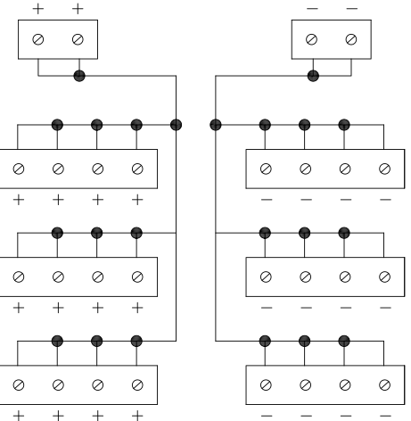
接線圖
