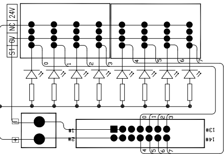
0241-C114K 接線圖
