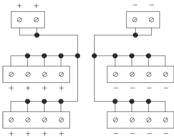
接線圖
