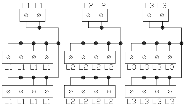
接線圖
