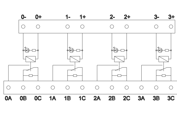
接線圖
