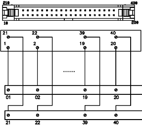
0241-C1XXS 接線圖
