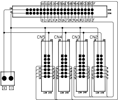
0241-C114K 接線圖
