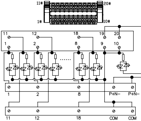
0241-C420LEDA 接線圖
