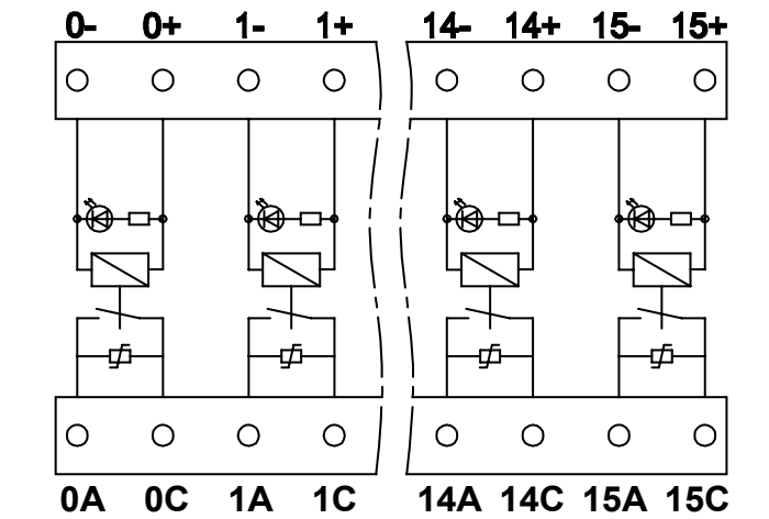
接線圖
