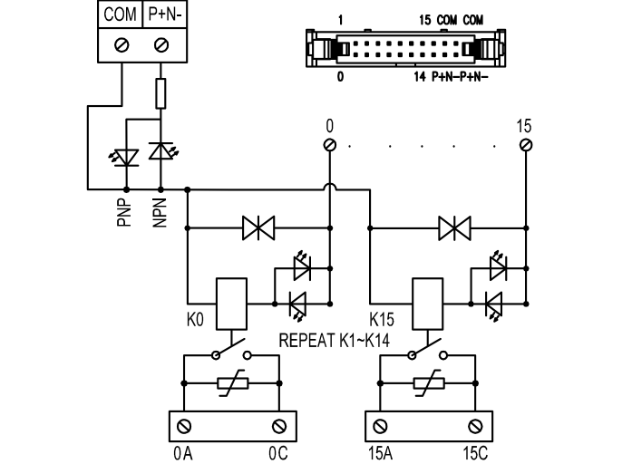
接線圖
