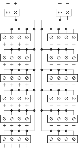
接線圖
