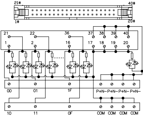
0241-C140LED 接線圖
