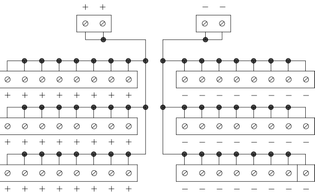
接線圖
