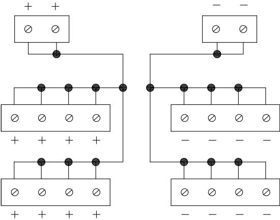
接線圖
