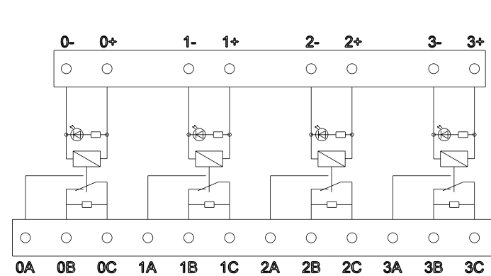
接線圖
