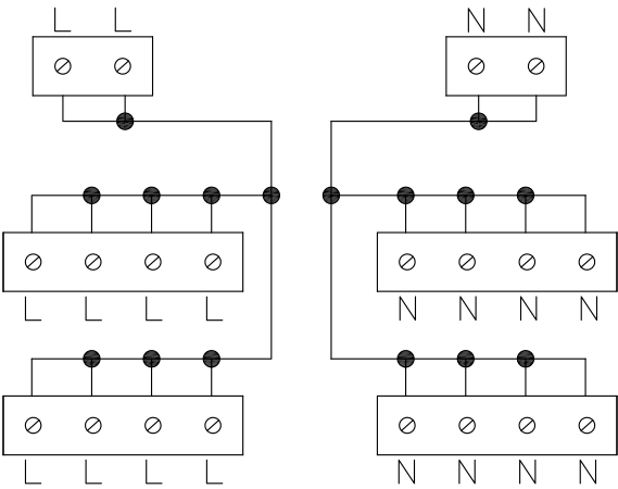
接線圖
