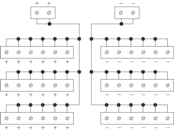
接線圖
