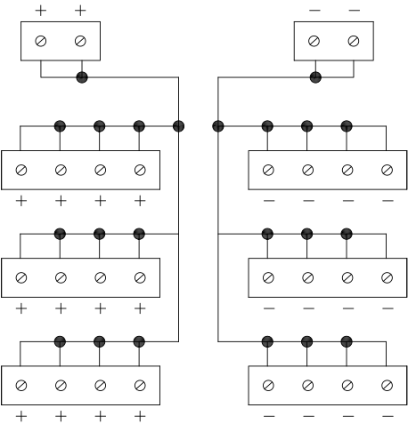
接線圖
