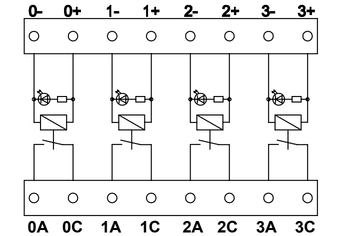
接線圖
