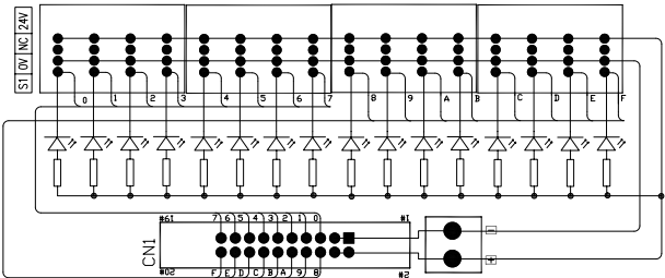
0241-C120K 接線圖
